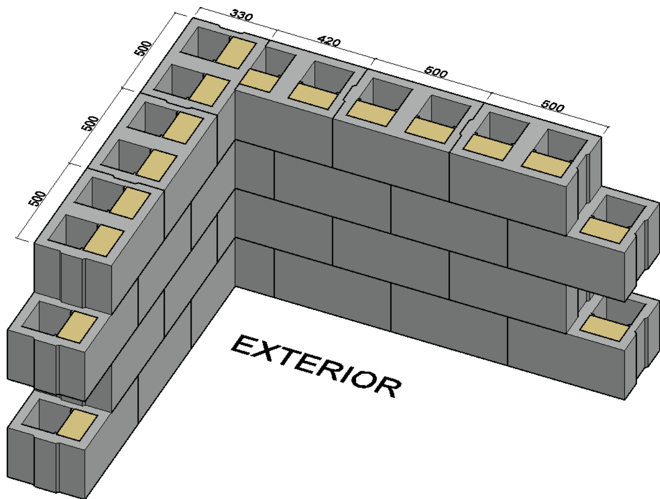
Dispunerea celui de al patrulea rând de blocuri Caloriblock
