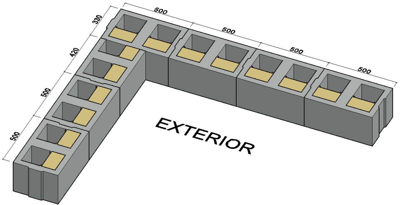
Dispunerea primului rând de blocuri Caloriblock
