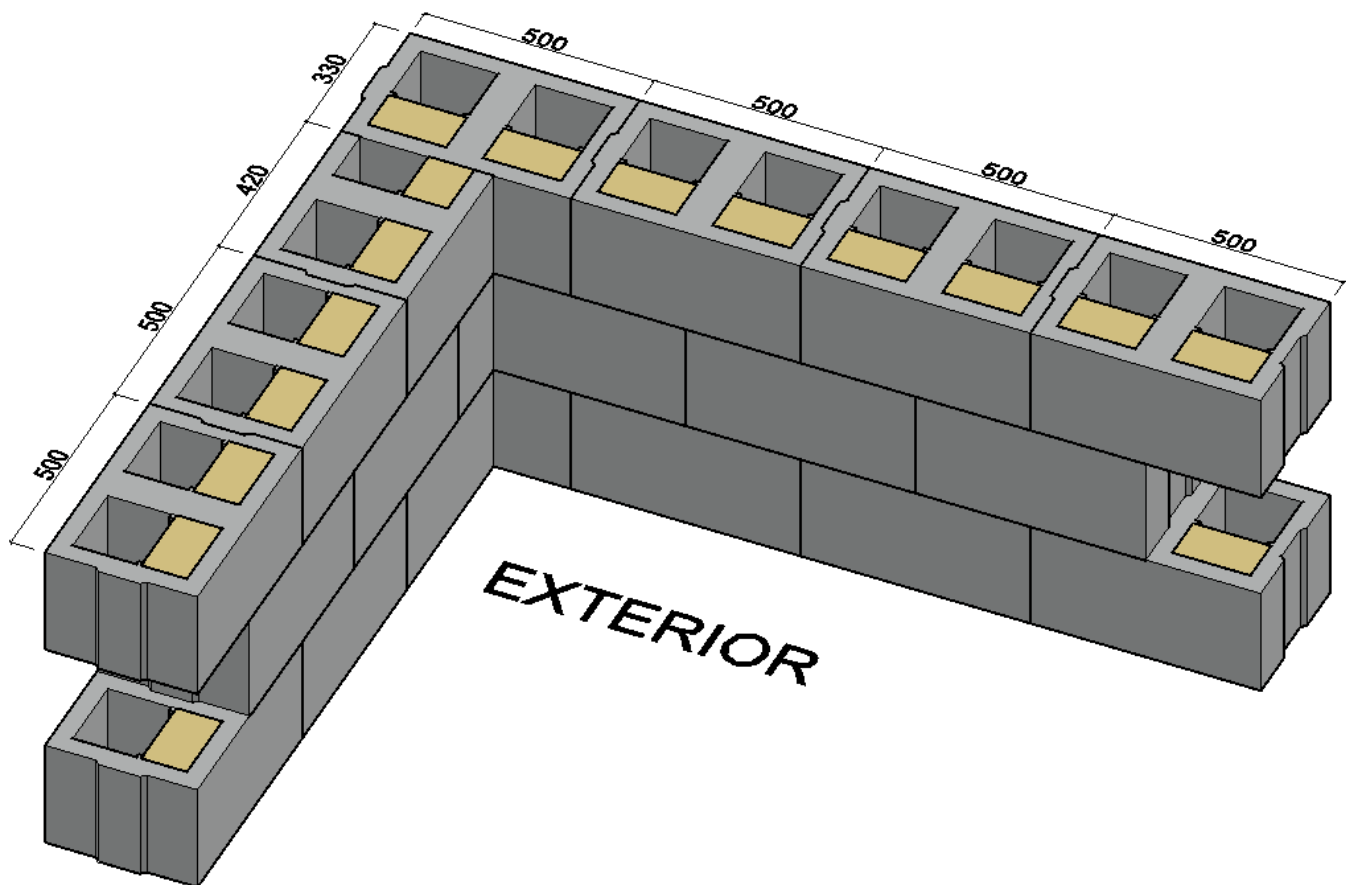
Dispunerea celui de al treilea rând de blocuri Caloriblock
