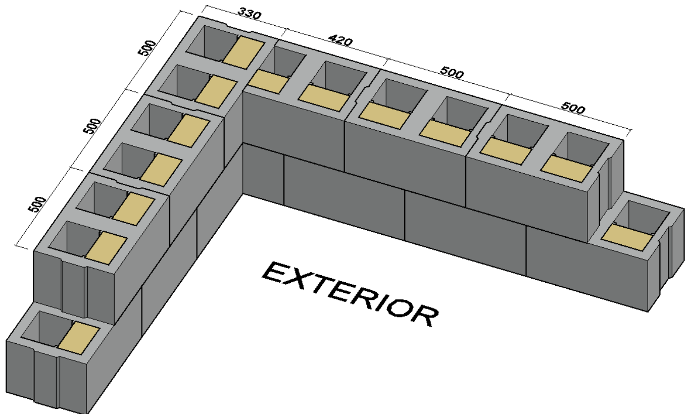
Dispunerea celui de al doilea rând de blocuri Caloriblock
